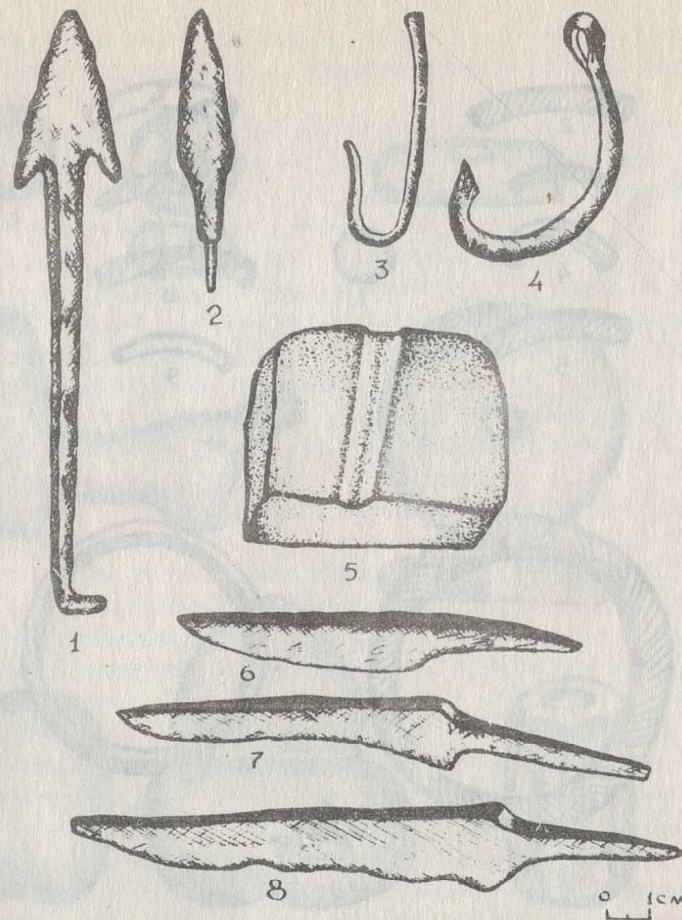
Рис. 7. Предметы кузнечного ремесла XI-XIII в.в. 1- наконечник дротика ; 2- наконечник стрелы ; 3-4- рыболовные крючки ; 5- точильный брусок ; 6-8- ножи .
