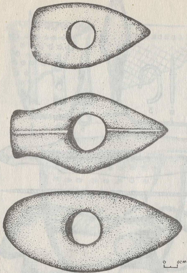
Рис. 2. Каменные топоры-молотки.
