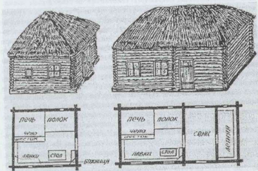
Жилая курная изба. Ливенский уезд. XIX век. Реконструкция Г. Рыжкина.
