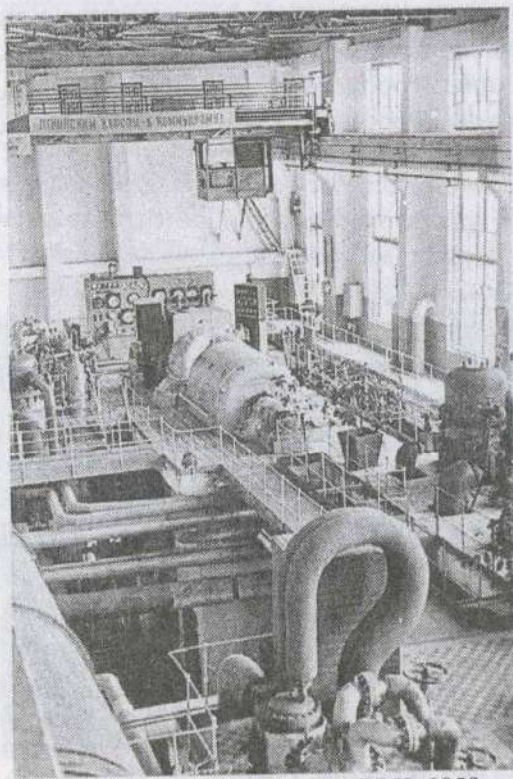
Турбинный зал Ливенской ТЭЦ. 1958 г.
